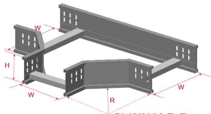
BL4/N20CA-T Tee
